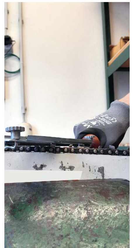
Abb. 8: Waagrechtes Auflegen der Feilenlehre; Foto: Andreas Löbnitz
