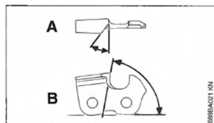
Abb. 4: Schärf- und Brustwinkel; aus: Bedienungsanleitung Stihl MS 261 - C
