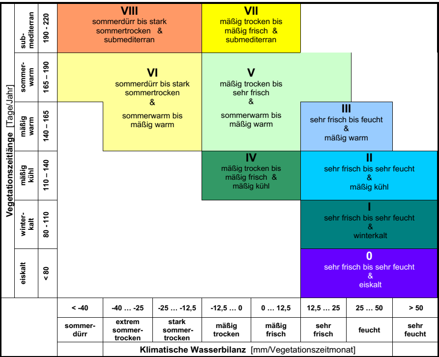
Abb. 2: Gliederungsrahmen der dynamischen Klimastufen
