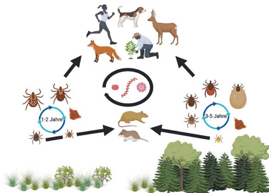
Schematische Darstellung der Entwicklungszyklen des Gemeinen Holzbocks (rechts) und der Wiesenzecke (links), deren Wirtstiere und bevorzugtes Habitat. Die zwischen Tieren und Menschen übertragbaren Erreger sind ebenfalls schematisch als Schraubenbakterium (Borrelien), Bakterium (Rickettsien, Anaplasma phagocytophilum ) und Virus (FSME-Virus) gezeigt; Grafik: Prof. Dr. Martin Pfeffer
